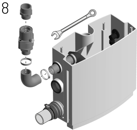
– Monter la sortie de pression
