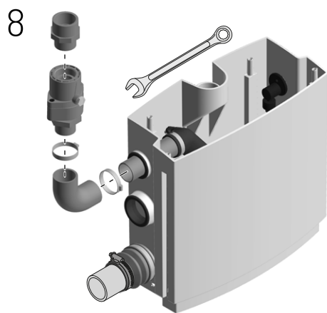
8 - Montaż odejścia tłocznego
